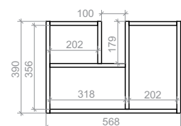
Ящик тумбы. Вид сверху
